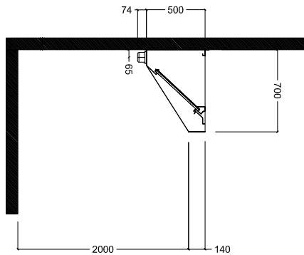
Boven aanzicht
